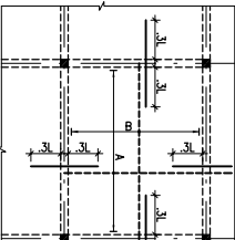
TYP. SLAB R/F DETAIL
