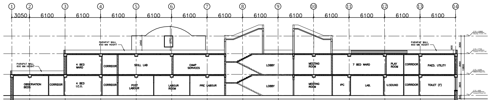
SECTION D-D
